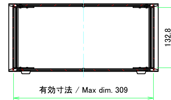
A-A ( 1 : 5 )
