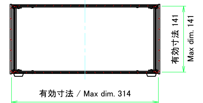
C-C ( 1 : 5 )
