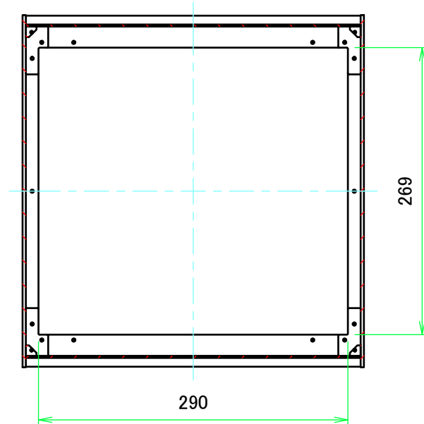
B-B ( 1 : 5 )
