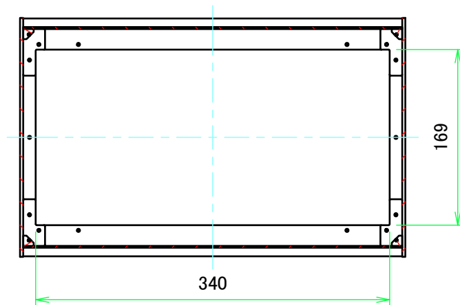
B-B ( 1 : 5 )
