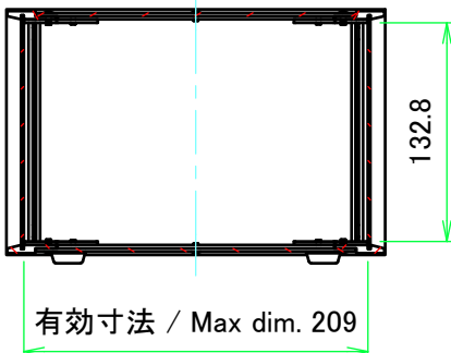
A-A ( 1 : 5 )
