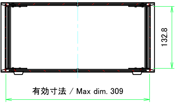
A-A ( 1 : 5 )
