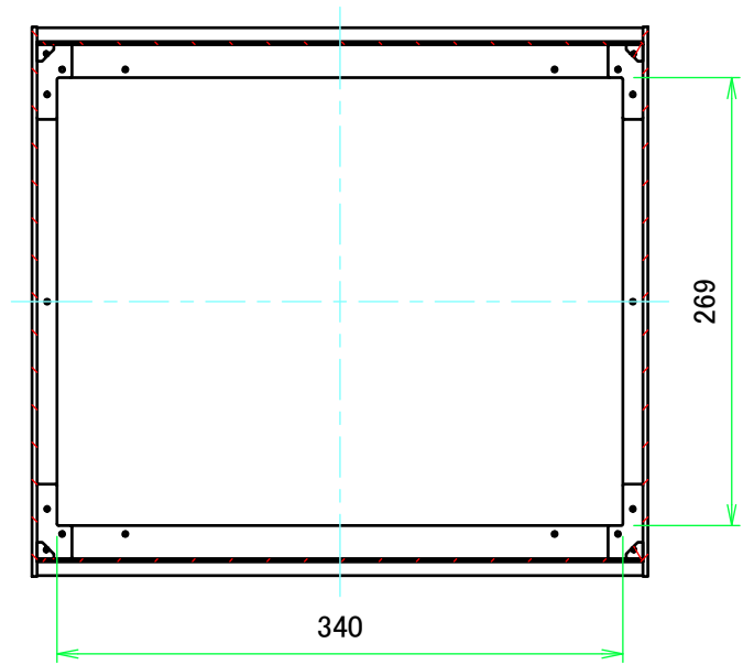
B-B ( 1 : 5 )
