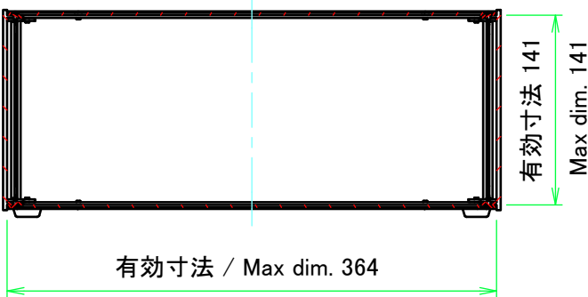
C-C ( 1 : 5 )
