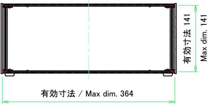
C-C ( 1 : 5 )
