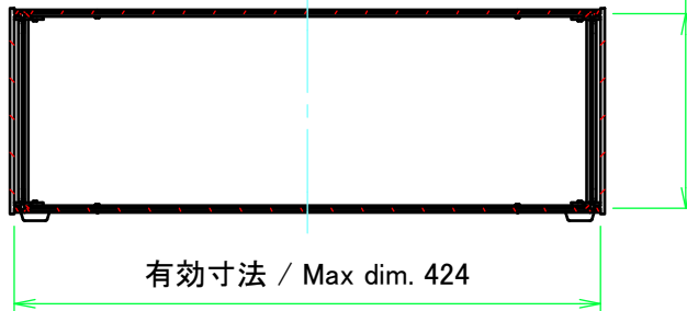
C-C ( 1 : 6 )
