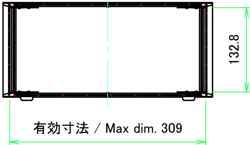
A-A ( 1 : 6 )
