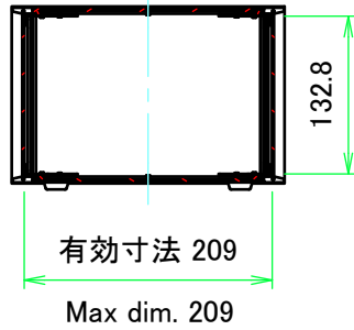
A-A ( 1 : 7 )
