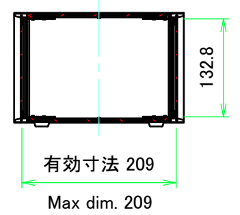
A-A ( 1 : 7 )
