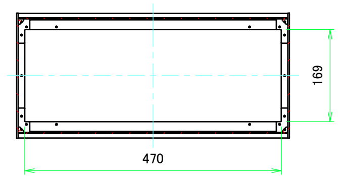
B-B ( 1 : 7 )
