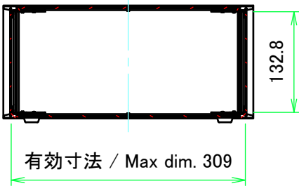
A-A ( 1 : 7 )
