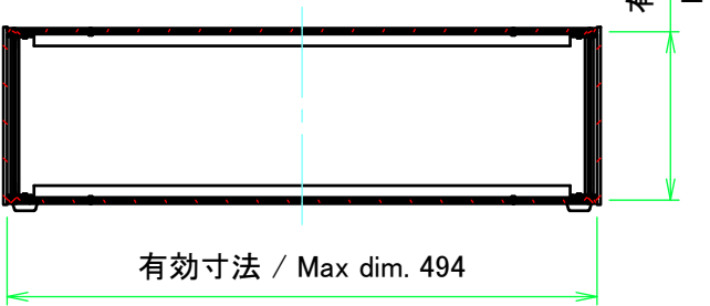
C-C ( 1 : 7 )
