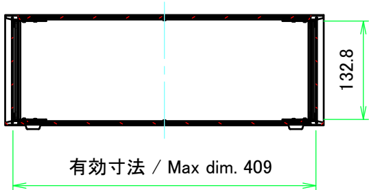
A-A ( 1 : 7 )
