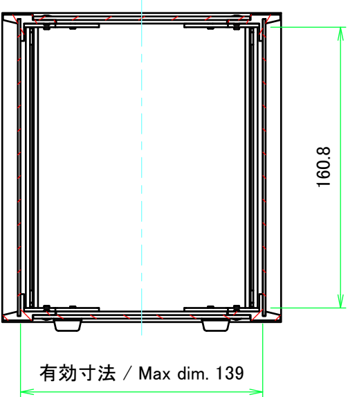
A-A (1:3)
