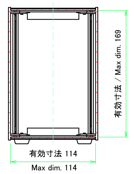
C-C ( 1 : 3 )
