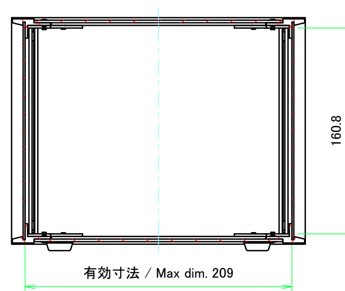
A-A ( 1 : 3 )
