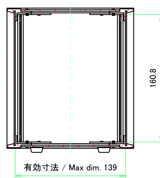
A-A ( 1 : 3 )
