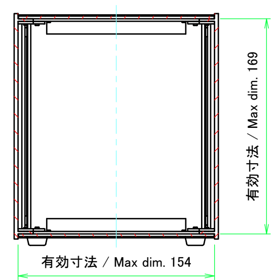
C-C ( 1 : 3 )
