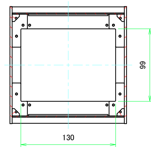
B-B ( 1 : 3 )
