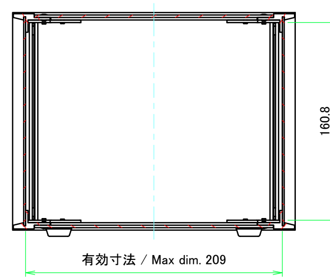
A-A (1:3)
