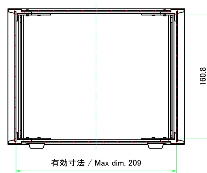
A-A (1:3)
