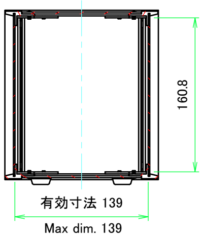
A-A ( 1 : 4 )
