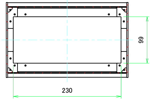
B-B ( 1 : 4 )
