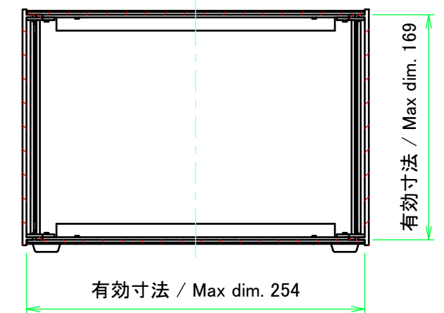
C-C ( 1 : 4 )
