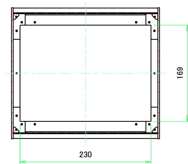
B-B ( 1 : 4 )
