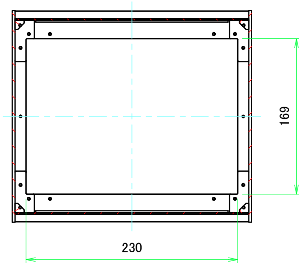
B-B ( 1 : 4 )
