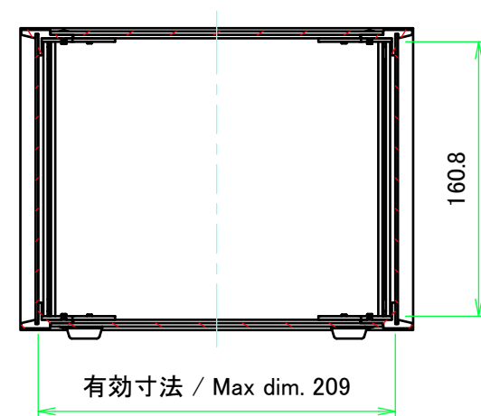
A-A ( 1 : 4 )
