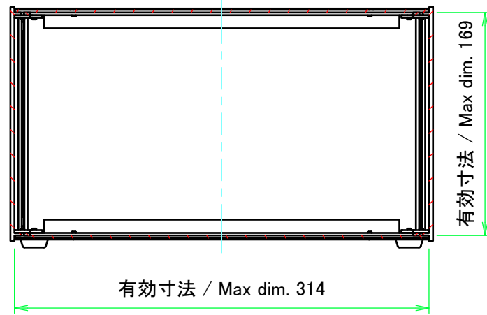
C-C ( 1 : 4 )
