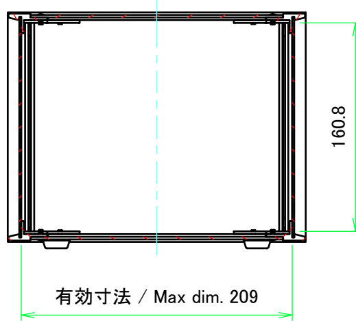
A-A ( 1 : 4 )
