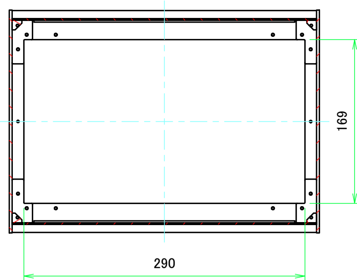
B-B ( 1 : 4 )
