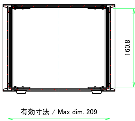
A-A ( 1 : 4 )
