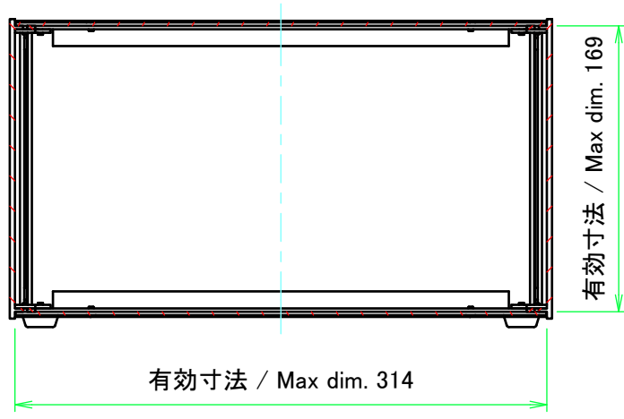
C-C ( 1 : 4 )
