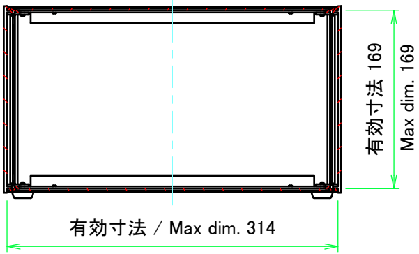
C-C ( 1 : 5 )
