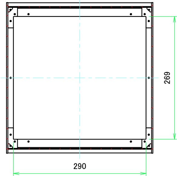
B-B ( 1 : 5 )
