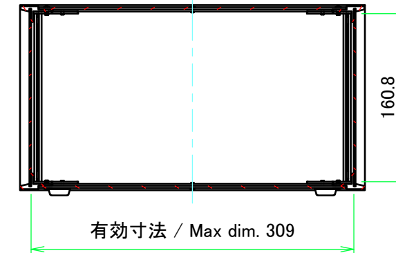
A-A (1:5)
