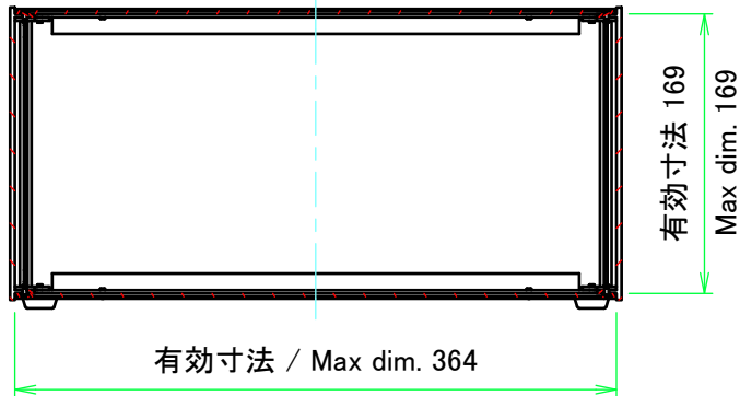
C-C ( 1 : 5 )
