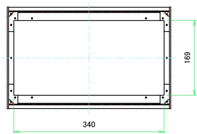
B-B ( 1 : 5 )
