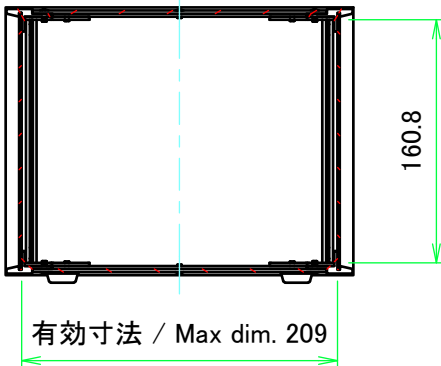
A-A ( 1 : 5 )
