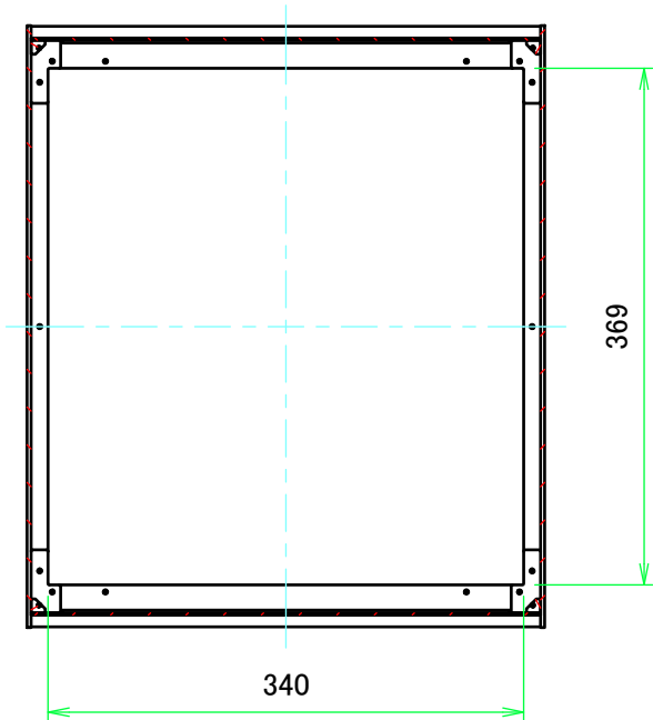
B-B ( 1 : 6 )
