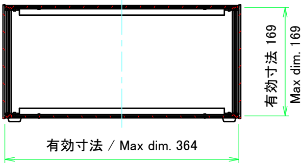
C-C ( 1 : 6 )
