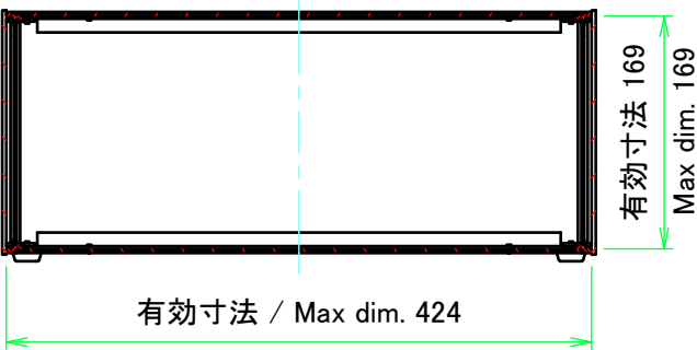
C-C ( 1 : 6 )
