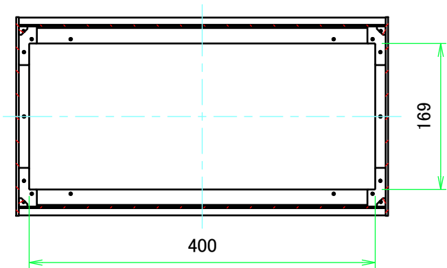
B-B ( 1 : 6 )
