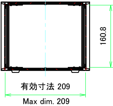
A-A ( 1 : 6 )
