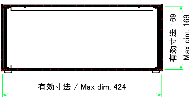
C-C ( 1 : 6 )
