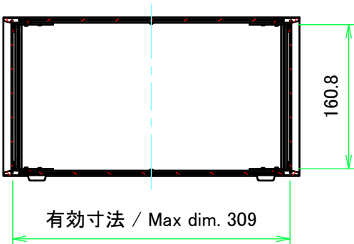
A-A ( 1 : 6 )
