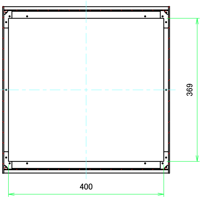
B-B ( 1 : 6 )
