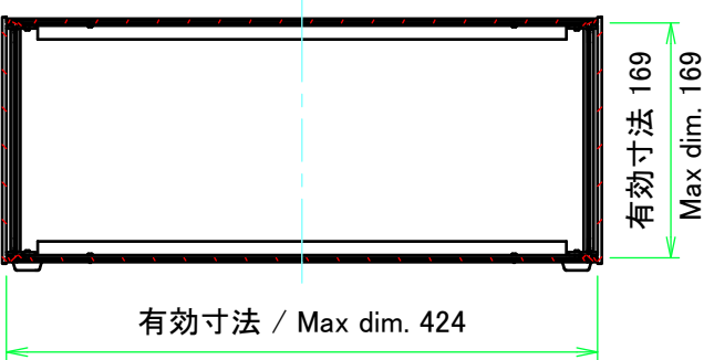
C-C ( 1 : 6 )
