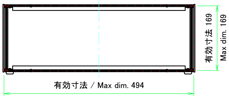
C-C ( 1 : 6 )
