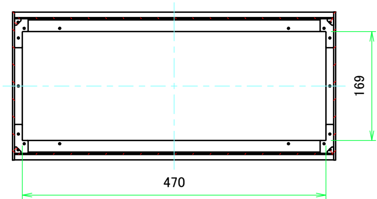
B-B ( 1 : 6 )
