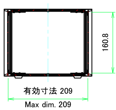
A-A ( 1 : 6 )
