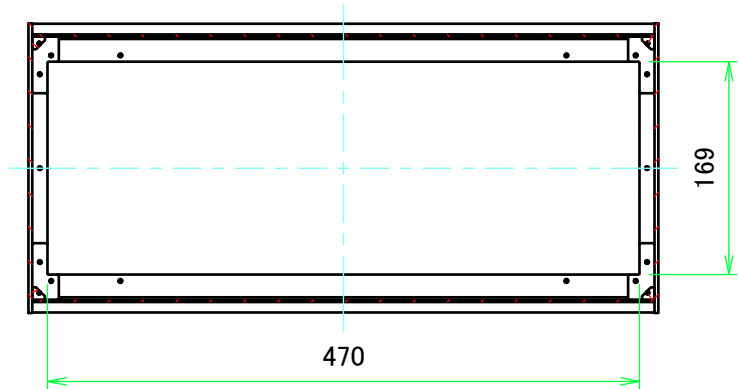
B-B ( 1 : 6 )
