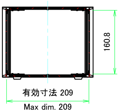
A-A ( 1 : 6 )
