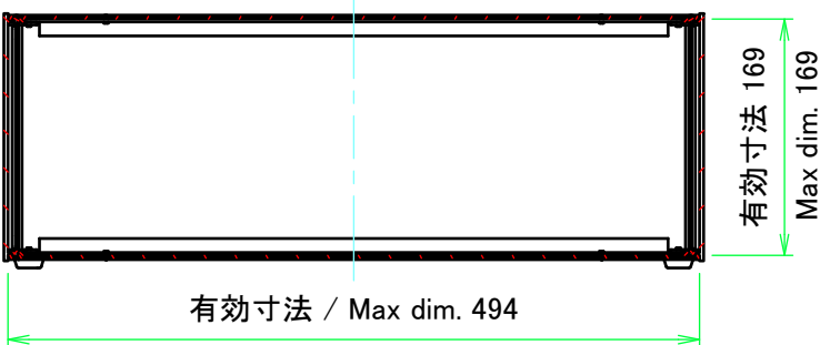
C-C ( 1 : 6 )
