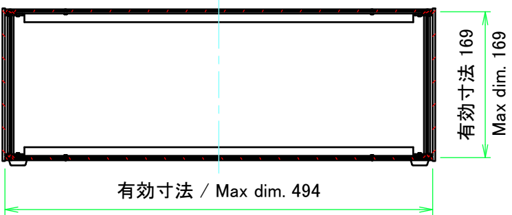
C-C ( 1 : 6 )
