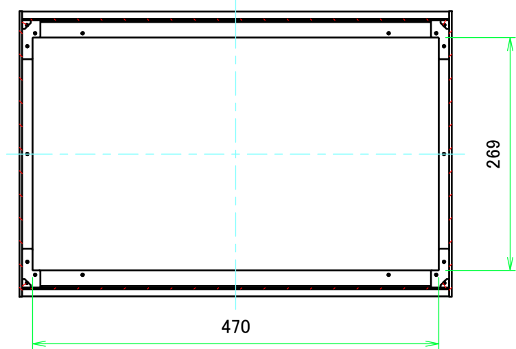
B-B ( 1 : 6 )
