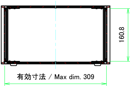
A-A ( 1 : 6 )
