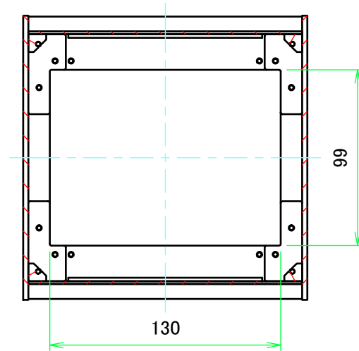
B-B ( 1 : 3 )
