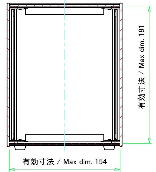
C-C ( 1 : 3 )
