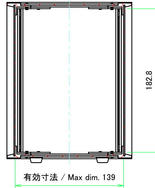
A-A ( 1 : 3 )
