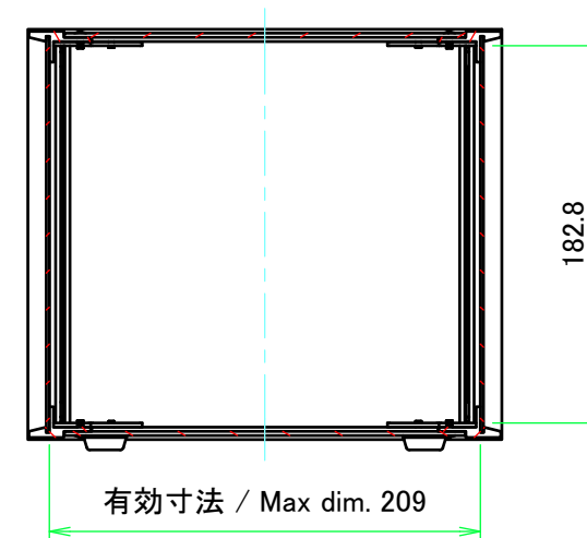
A-A ( 1 : 4 )
