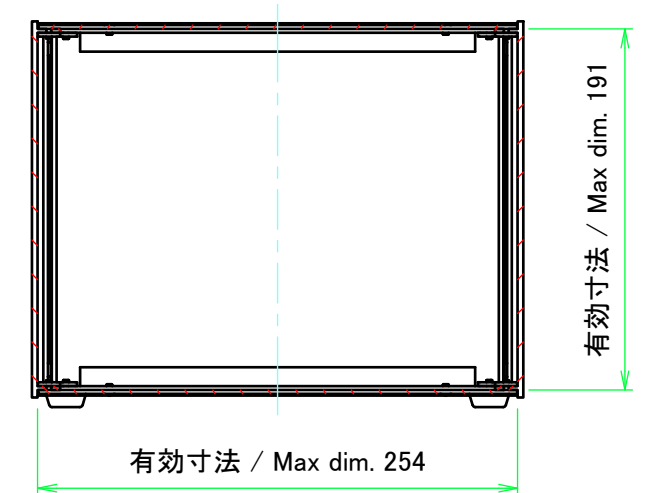
C-C ( 1 : 4 )
