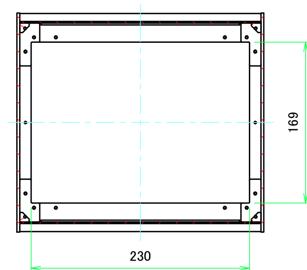
B-B ( 1 : 4 )
