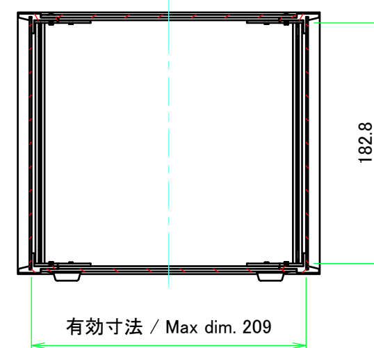
A-A ( 1 : 4 )
