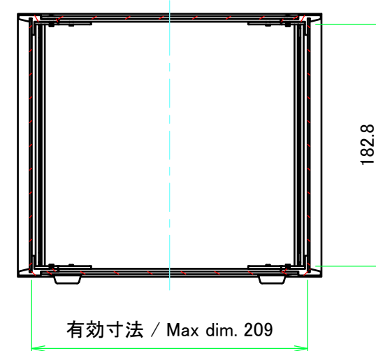
A-A ( 1 : 4 )
