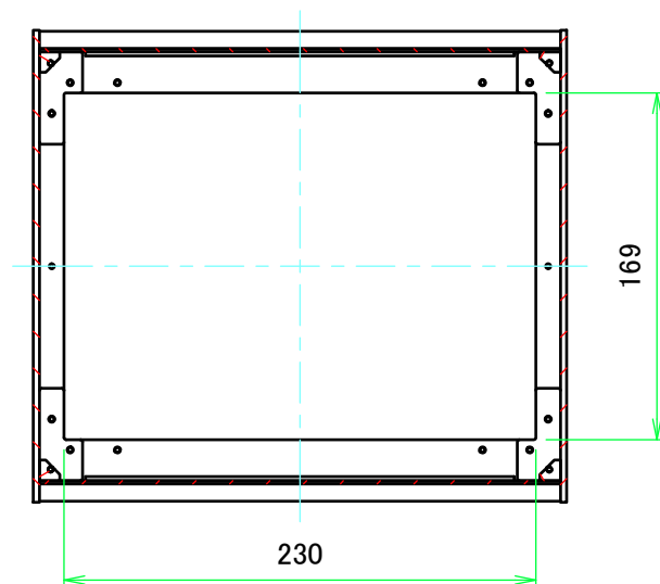
B-B ( 1 : 4 )
