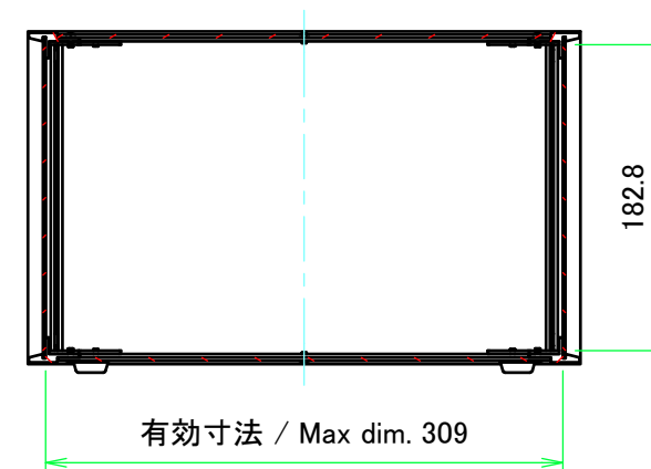
A-A (1:5)
