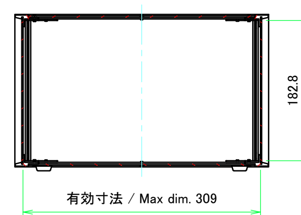
A-A (1:5)
