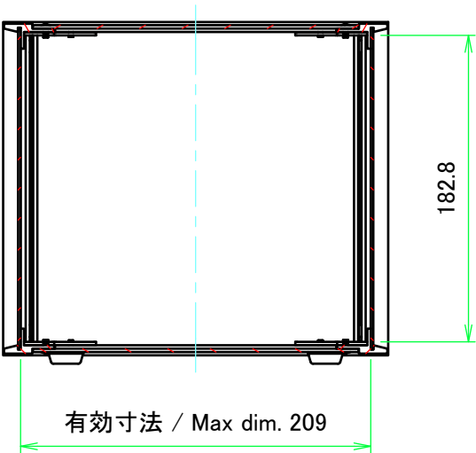
A-A ( 1 : 4 )
