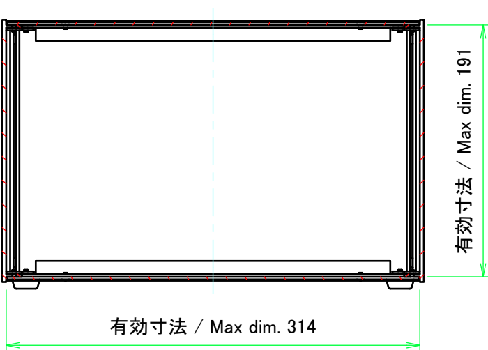
C-C ( 1 : 4 )
