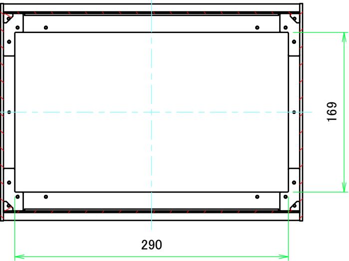
B-B ( 1 : 4 )
