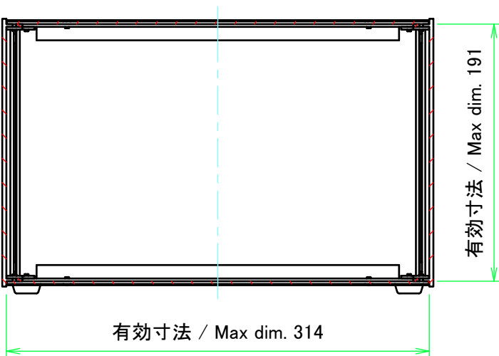
C-C ( 1 : 4 )
