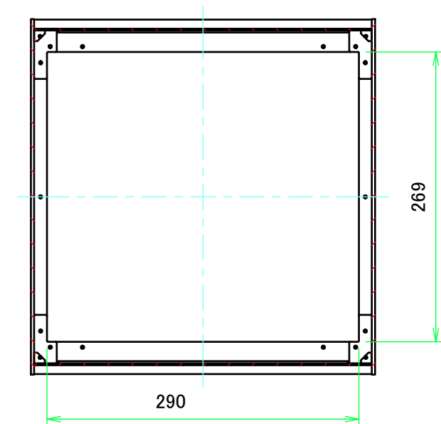
B-B ( 1 : 5 )
