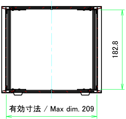
A-A (1:5)
