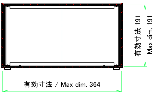
C-C ( 1 : 6 )
