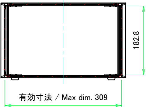
A-A ( 1 : 6 )
