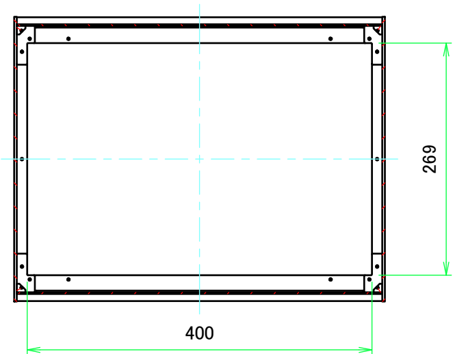
B-B ( 1 : 6 )
