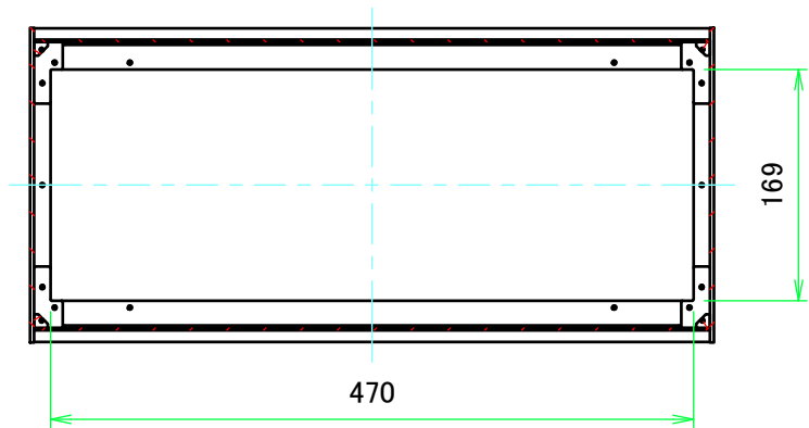
B-B ( 1 : 6 )
