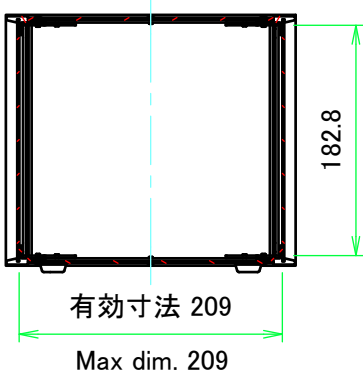
A-A ( 1 : 6 )
