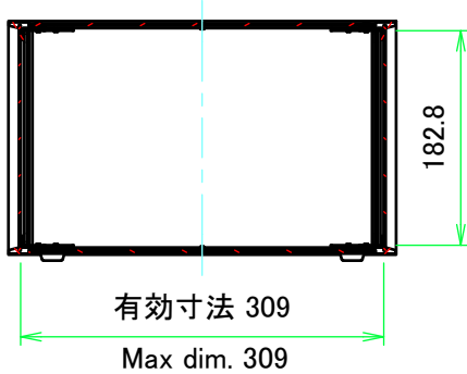
A-A ( 1 : 7 )
