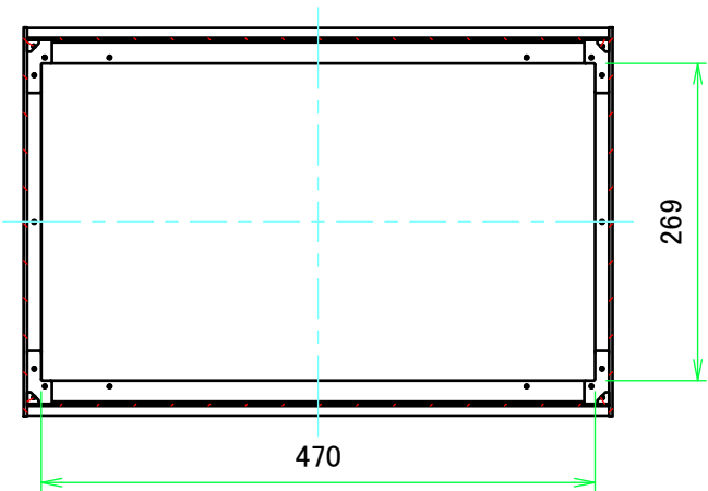
B-B ( 1 : 7 )
