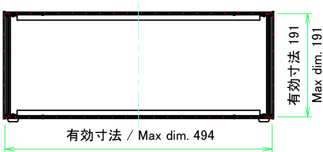
C-C ( 1 : 7 )
