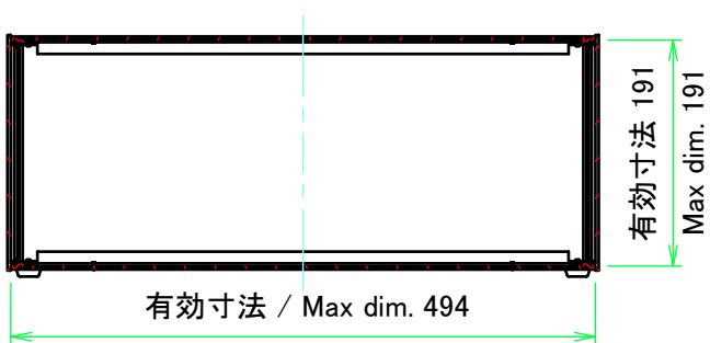
C-C ( 1 : 7 )
