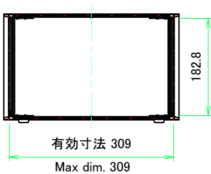
A-A ( 1 : 7 )
