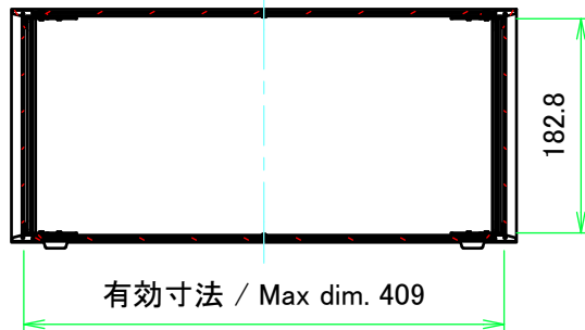
A-A (1:7)
