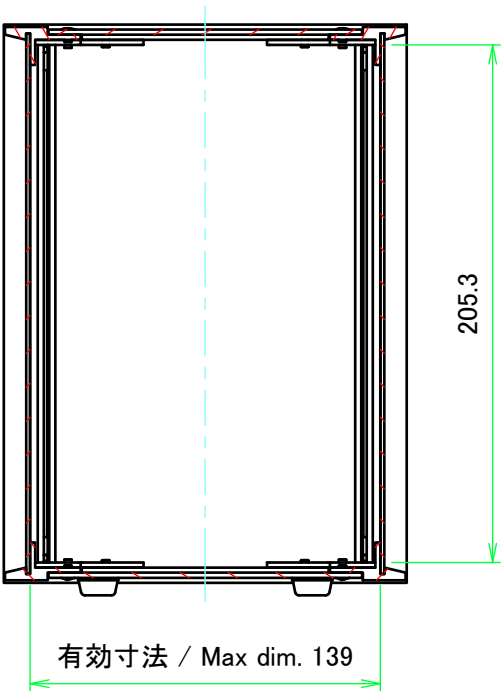
A-A (1:3)
