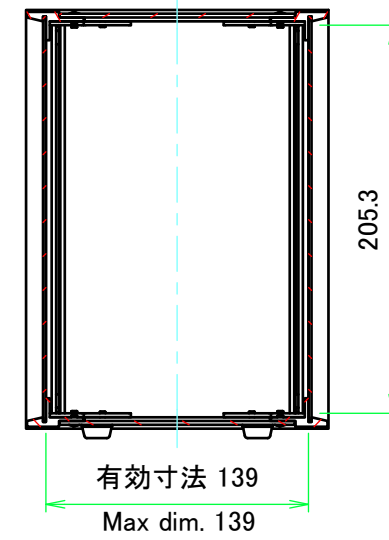
A-A (1:4)
