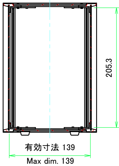
A-A ( 1 : 4 )
